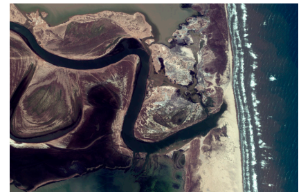
Figura 4. Imagen del satélite del Río Grande/Río Bravo en el Golfo de México.
