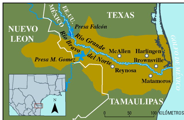
Figura 2. Área del estudio.
