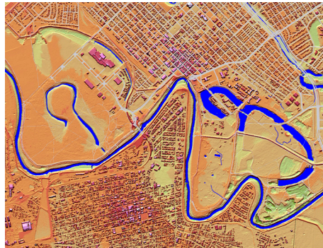
Figura 3. Modelo digital de alta resolución de la elevación.
